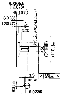
• Type USASEM-15AC2K* Type USASEM-15AC2KB†
