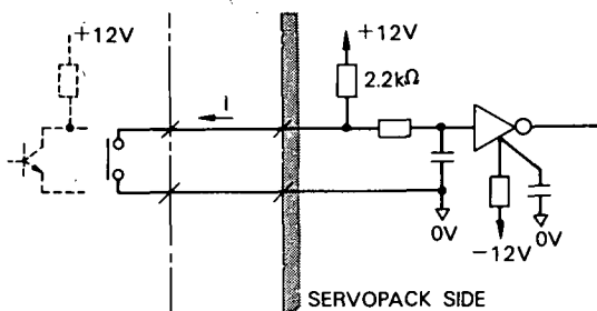
Fig. 6.3 Input Circuit (1)
